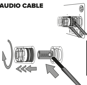
AUDIO CABLE
